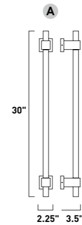
E21683-BK, -GLD, -PC, -SN Wall Mount
