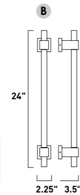
E21682-BK, -GLD, -PC, -SN Wall Mount
