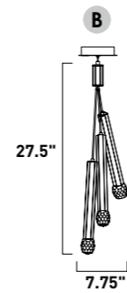
E23343-122BK, -122GLD Pendant
