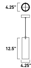
E21184-05GM, -54BK, -54SN, -118SN, -142GM Pendant
