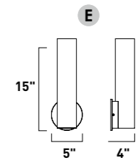
E21180-05GM, -54BK, -54SN, -118SN, -142GM Wall Mount
