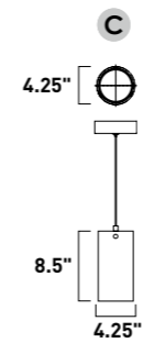
E21181-05GM, -54BK, -54SN, -118SN, -142GM Mini Pendant
