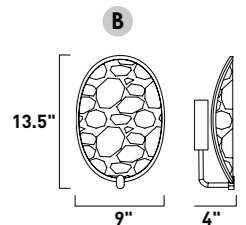
E24970-BCN, -PC Wall Mount
