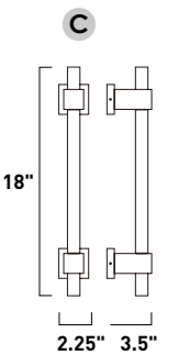
E21681-BK, -GLD, -PC, -SN Wall Mount
