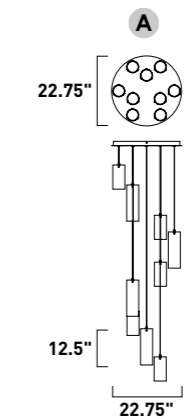
E21189-05GM, -142GM Pendant
